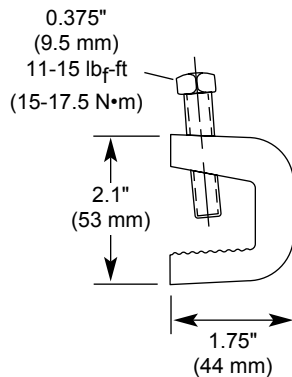
31768A stainless steel acero inoxidable acier inoxydable rostfreier Stahl aço inoxidável 不锈钢
