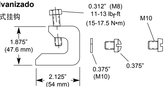
242774/ 242774-M (metric) galvanized steel acero galvanizado acier galvanisé verzinkter Stahl aço galvanizado 咔哒式挂钩
